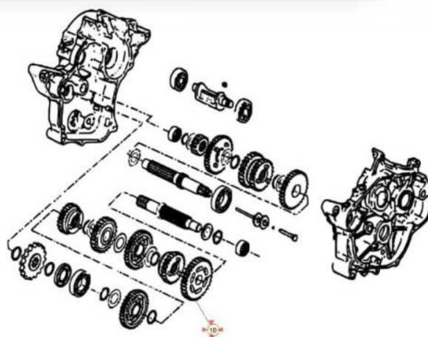
Scatola cambio esplosa
